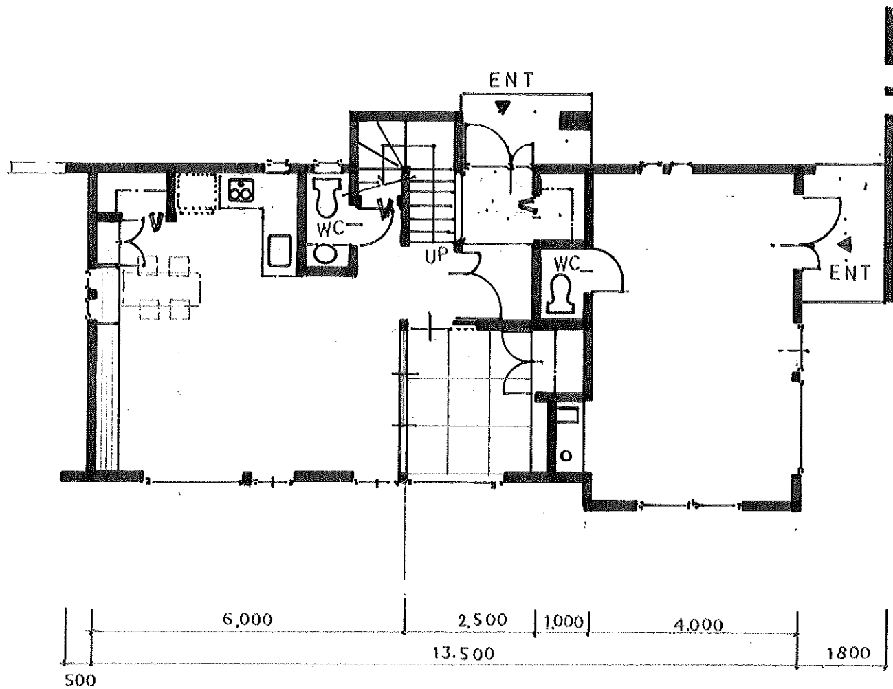
1 階平面図 1:100
