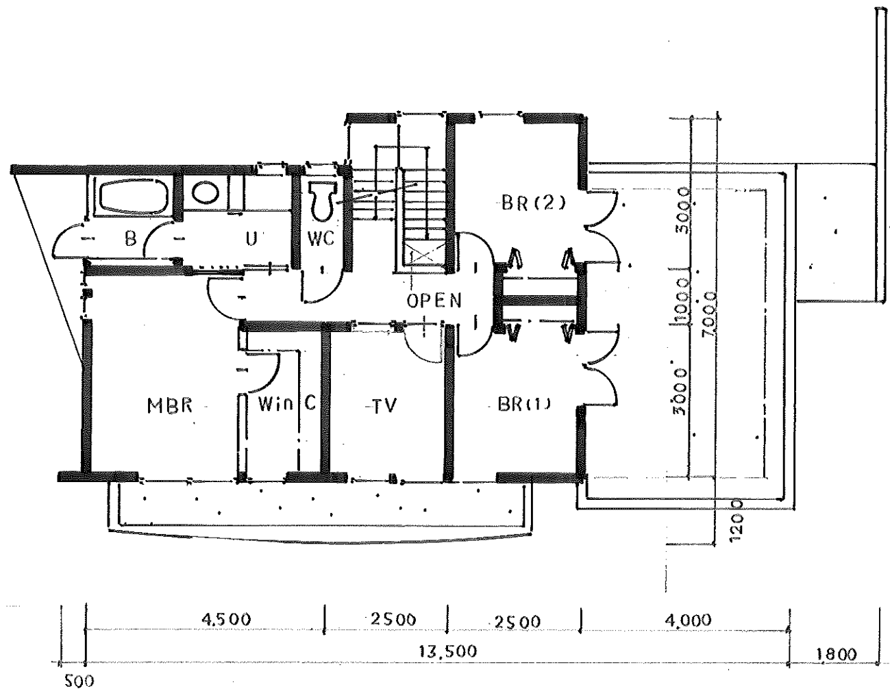
S-1:100 2 樓 平 面 圖
