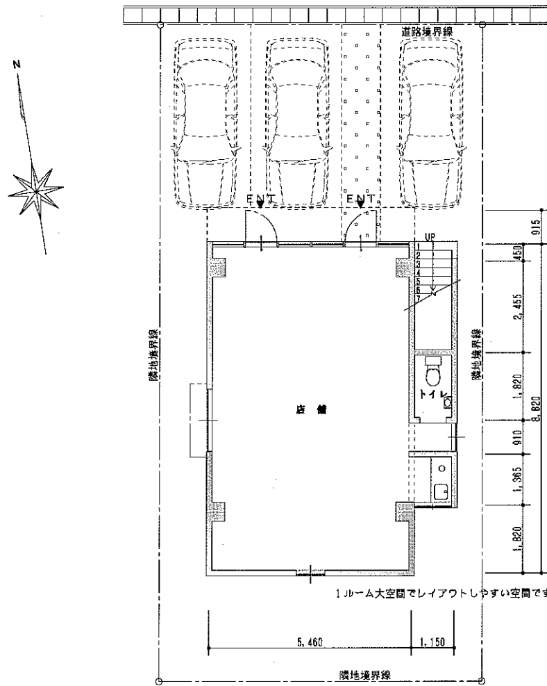
1階 平面図
